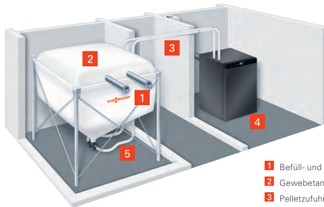
Pelletsilo (Gewebetank) mit Zuführung zum Pelletkessel durch Vakuum-Saugsystem
