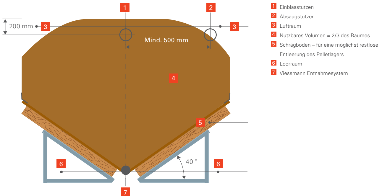
Lagerraum mit Schrägboden
