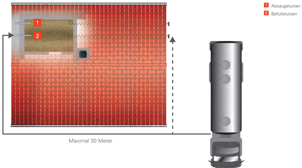
Lage des Pelletlagerraumes
