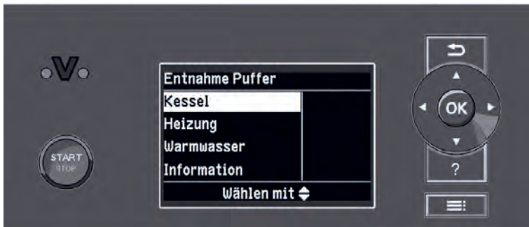
Die Regelung Ecotronic mit mehrzeiligem, beleuchtetem Display und Klartextanzeige sowie vereinfachter Inbetriebnahme (Inbetriebnahmeassistent) durch Plug-and-Work-Funktion
