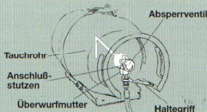
Abb. 2 Anschluß einer Treibgasflasche
