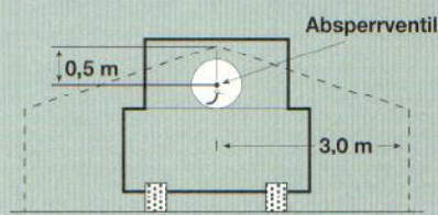
Abb. 1 Schutzbereich beim Abstellen von treibgasbetriebenen Fahrzeugen
